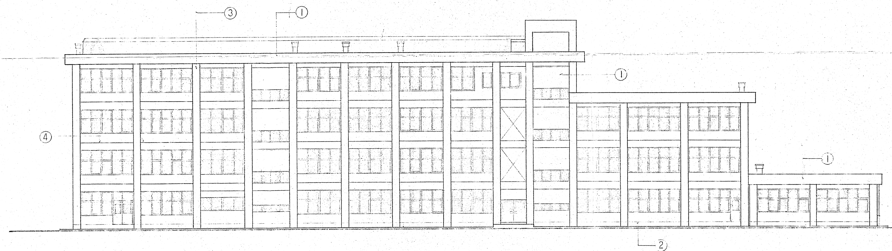
内部南立面図 S=1:200
