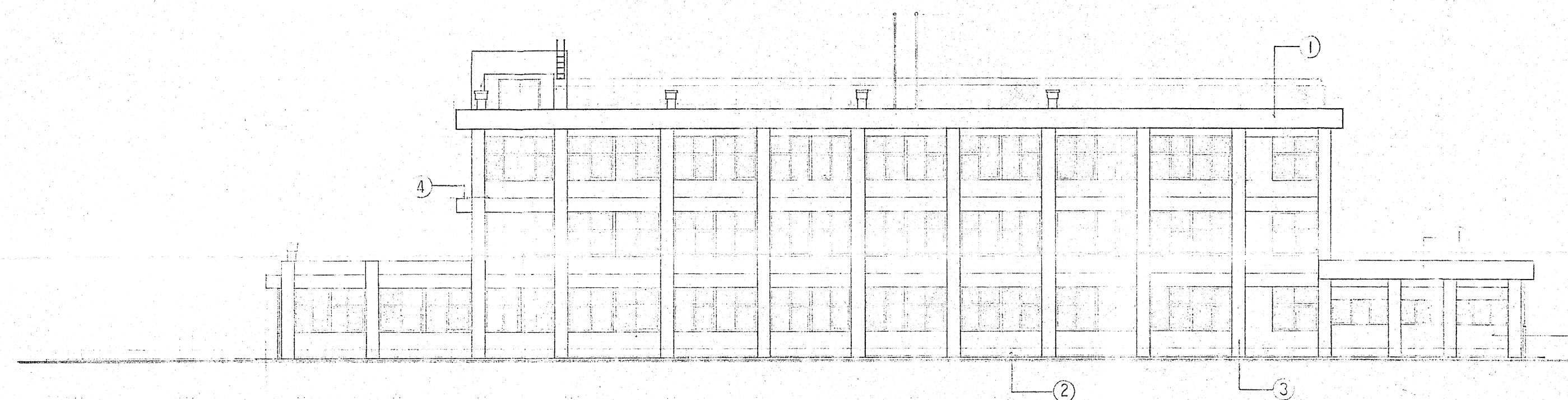
南立面图 3-1:200
