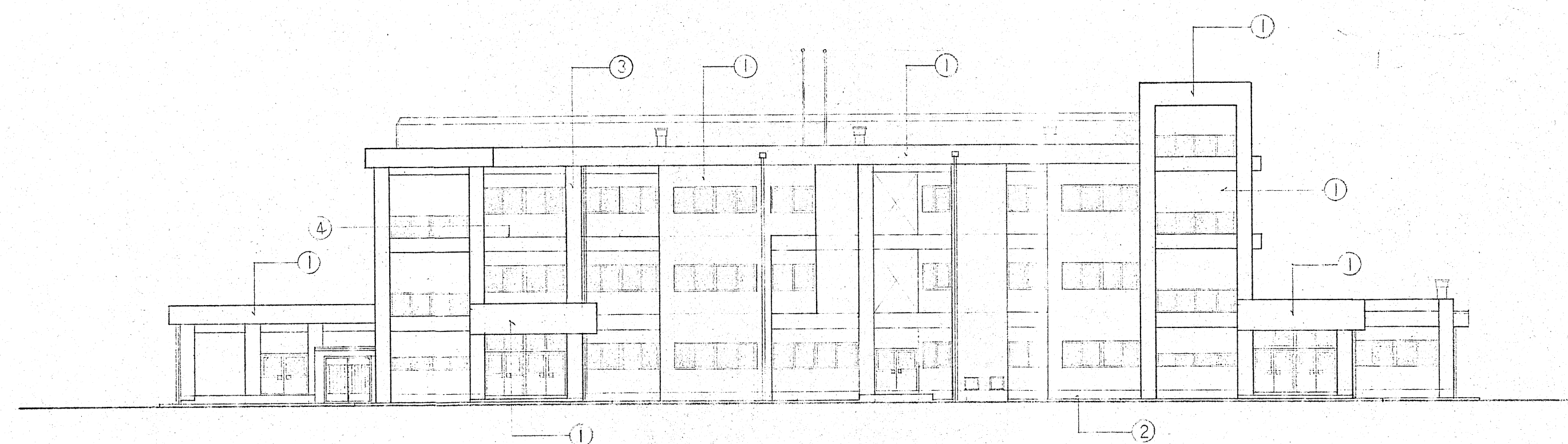
内部北立面図 S=1:200
