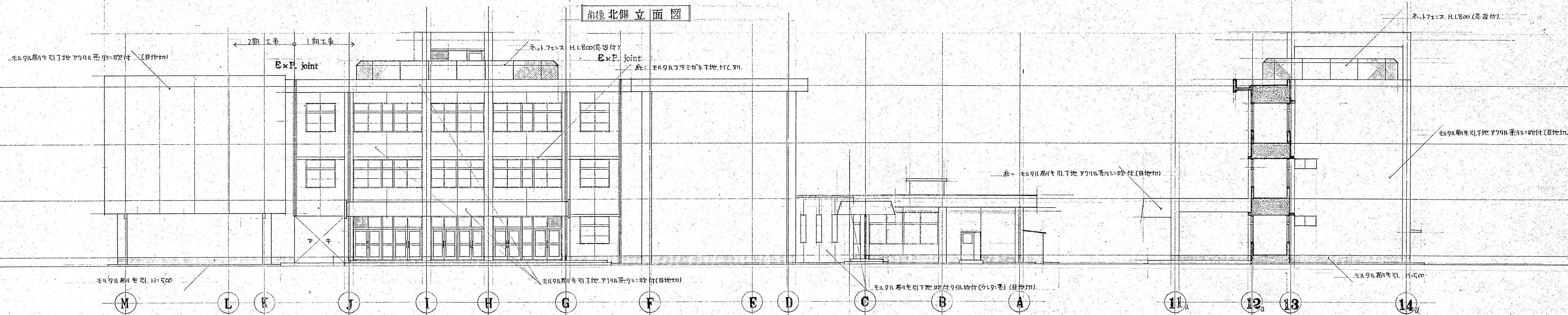
側面北側立面図
