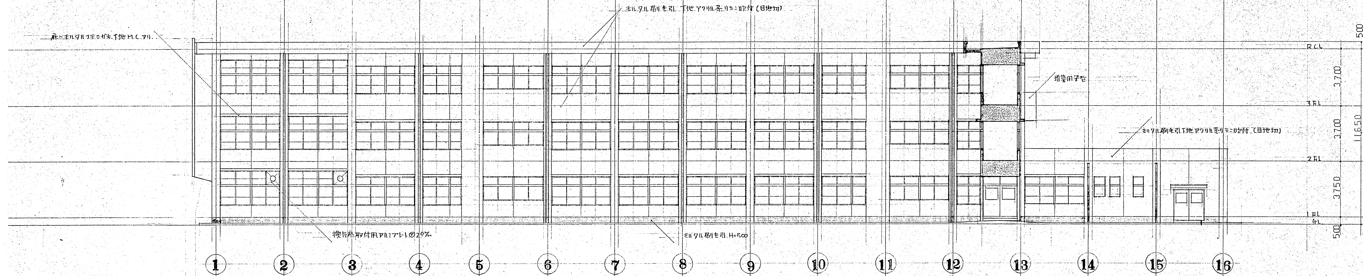
正面北側立面図
