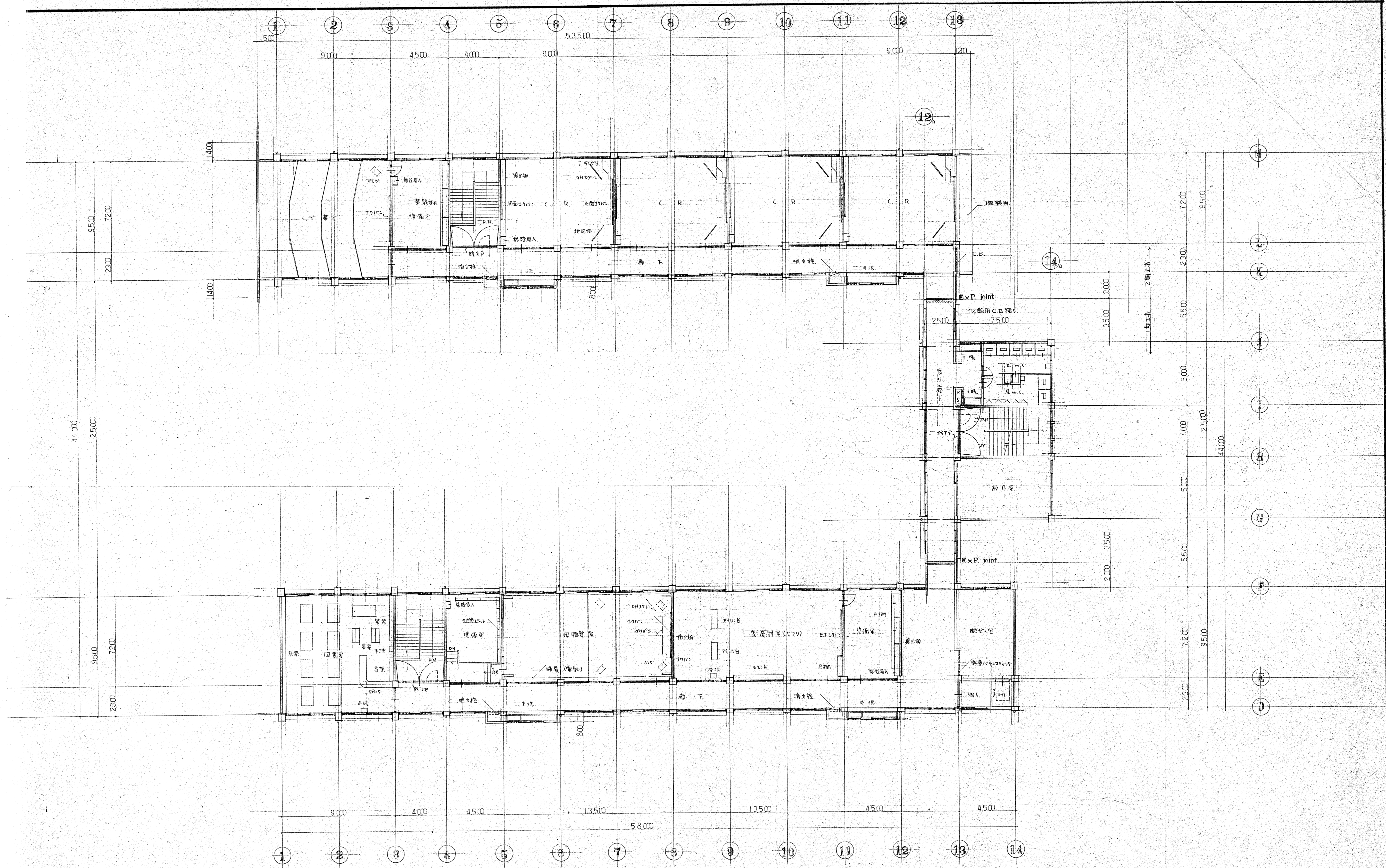
3階平面図 S=1:150
